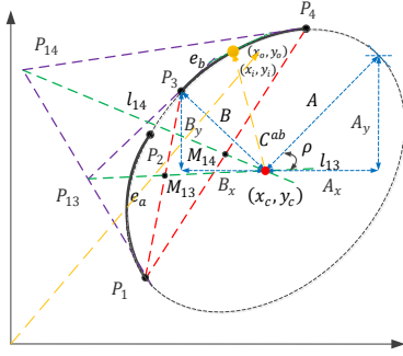
Fig. 9. Geometric schematic of parameter estimation.
